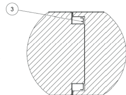
Vista detalle A machihembrado E: 1:20 E: 1:2
