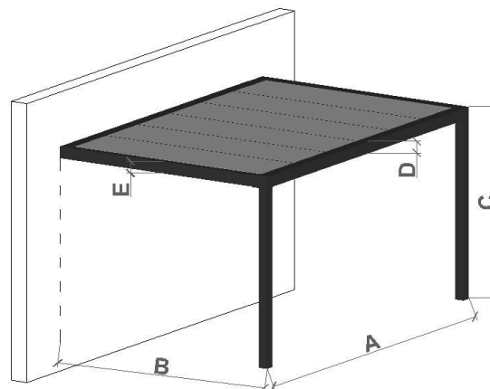
- 2 columnas perpendicular pared -
