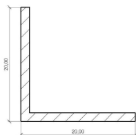
E0111- 19011 - ANGULO 20x20x1.5
